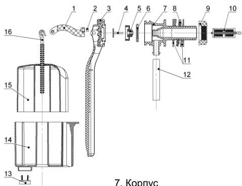
Рис. 1 - Клапан впуска (боковая подводка)
